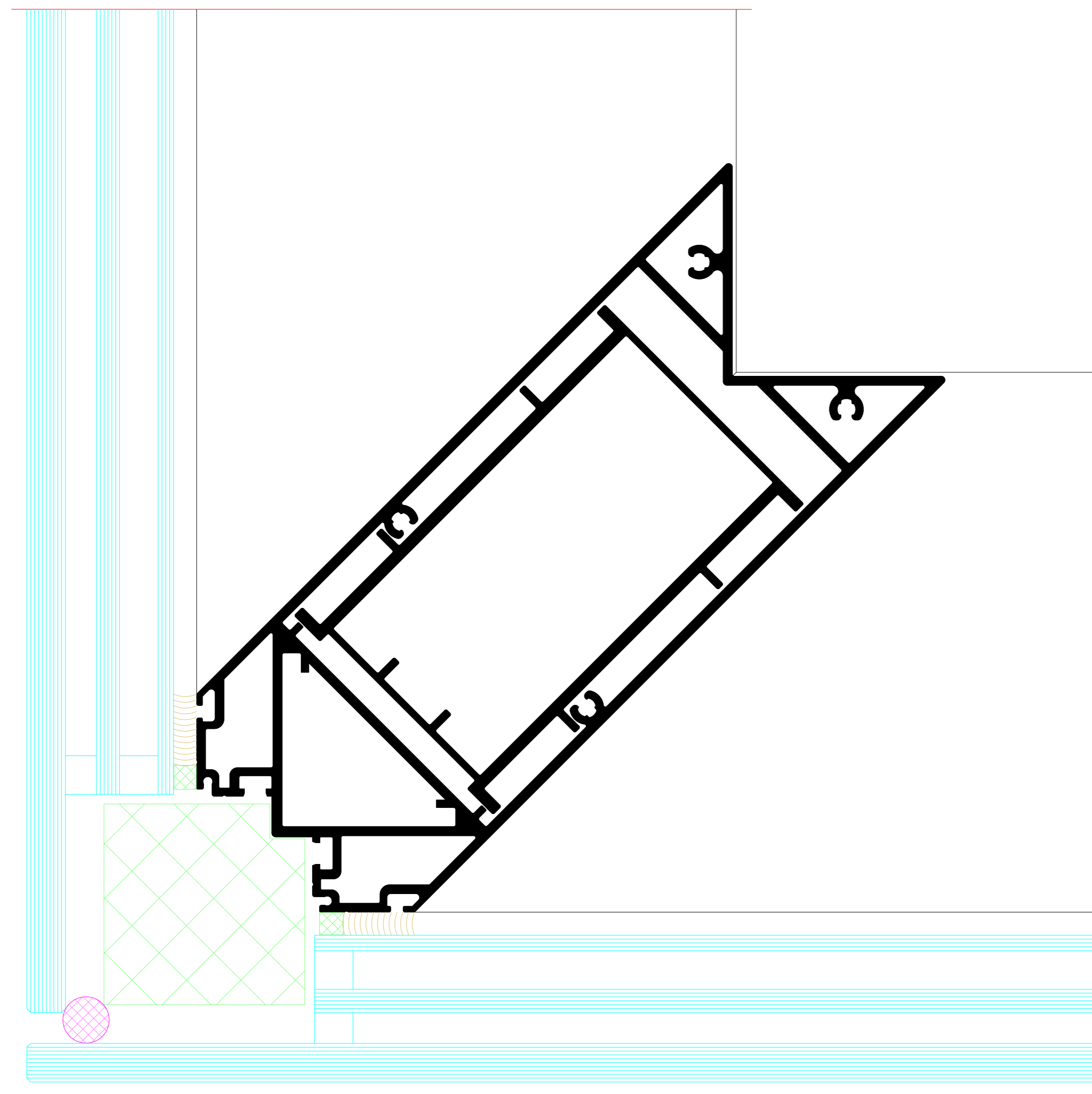
Horizontalschnitt durch AF UDC 80 SG 90°-Außenecke Horizontal section detail through AF UDC 80 SG outer corner
