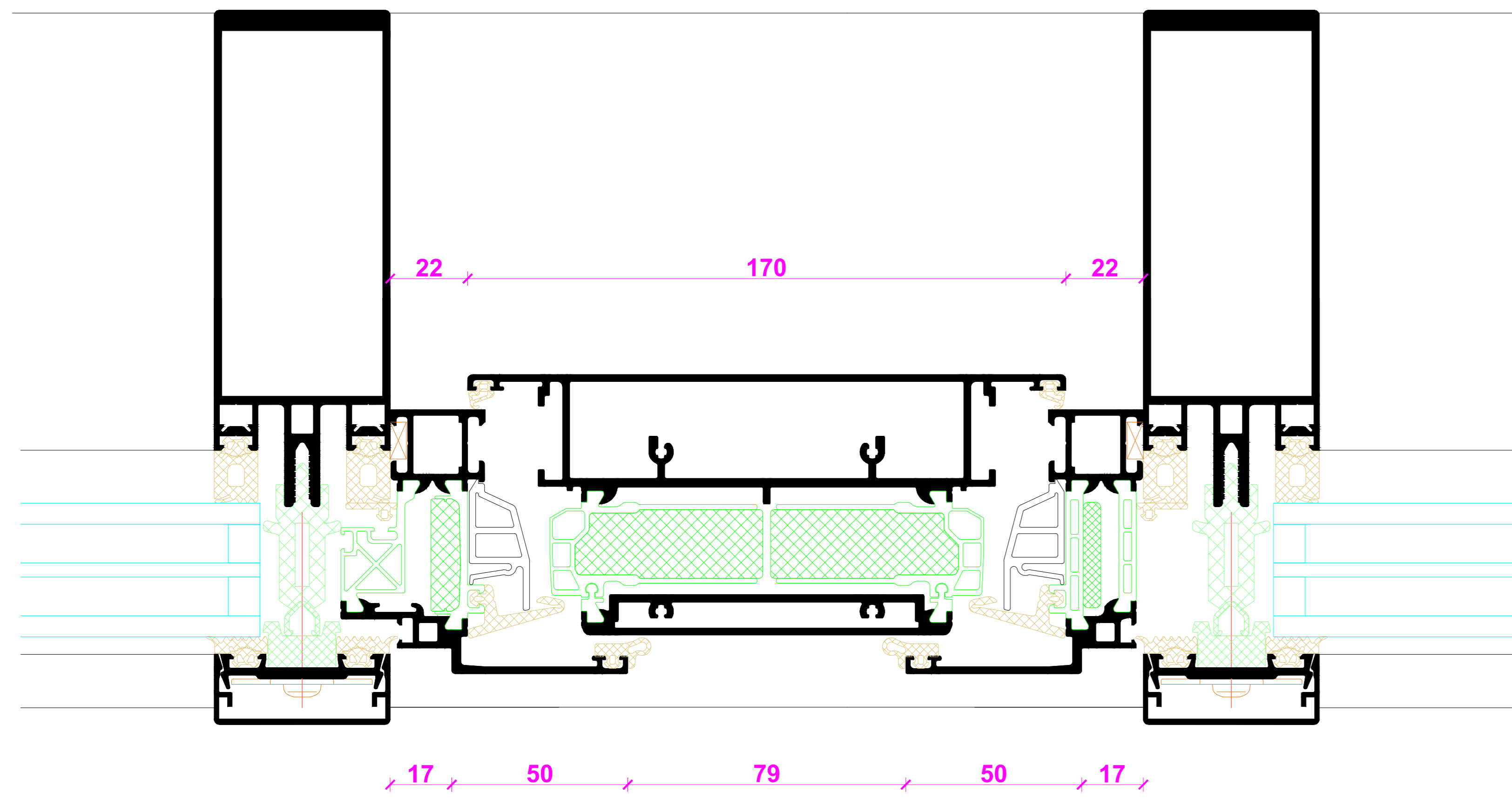
Flügel Aufschlagend/ AWS 90 VV.SI+ 170 mm Innenansicht / Außen flächenbündig
