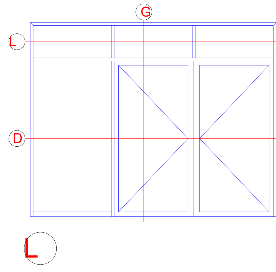
Zweiflügelige Tür mit Festfeld und Oberlicht Double-leaf door with fixed light and toplight
