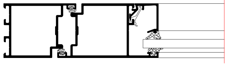
Flügelprofil Vent profile
