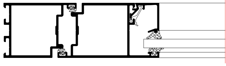
Blendrahmenprofil Outer frame profile
