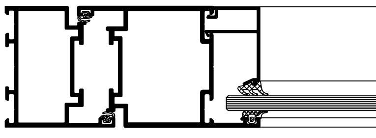
Flügelprofil Leaf profile
