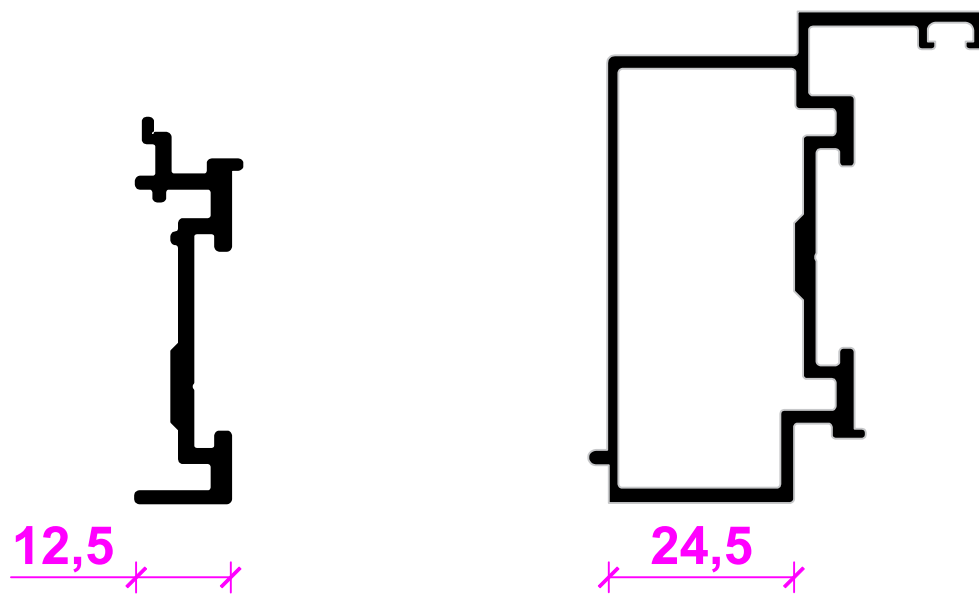
Anschlagprofil 25 Rebate profile 25
