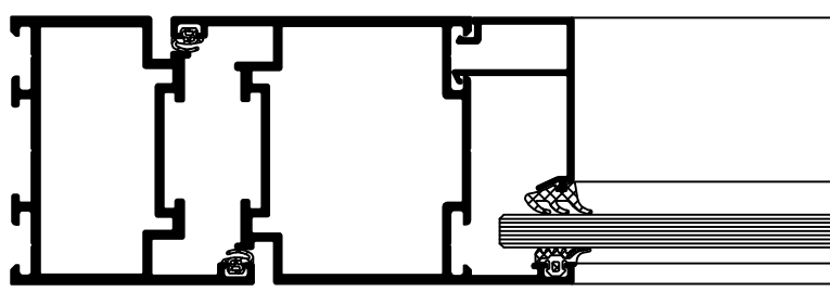
Blendrahmenprofil Outer frame profile
