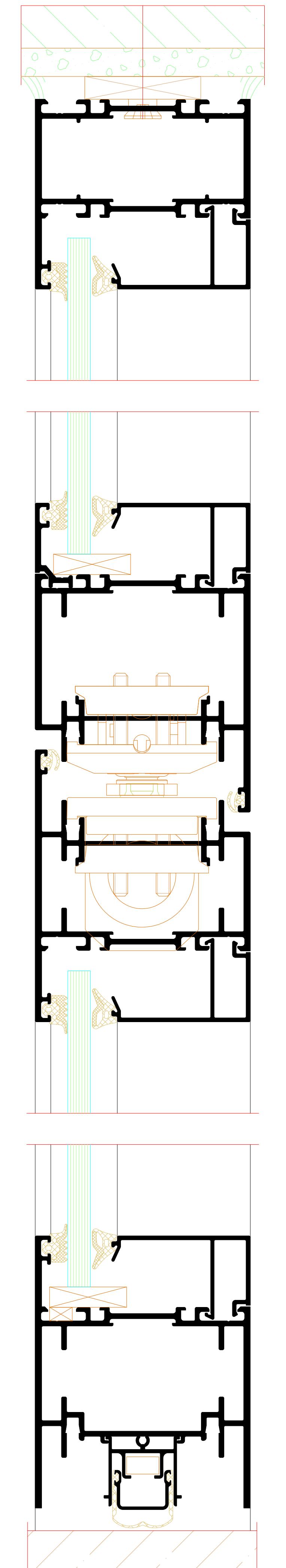
Türflügel mit Oberlicht Door leaf with toplight
