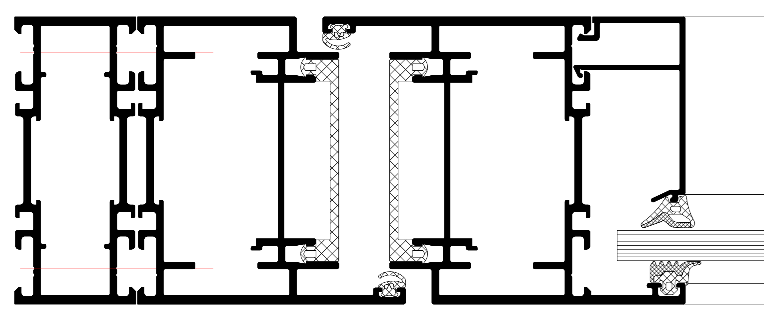
Blendrahmenverbreiterungsprofil Blendrahmenverbreiterungsprofil
