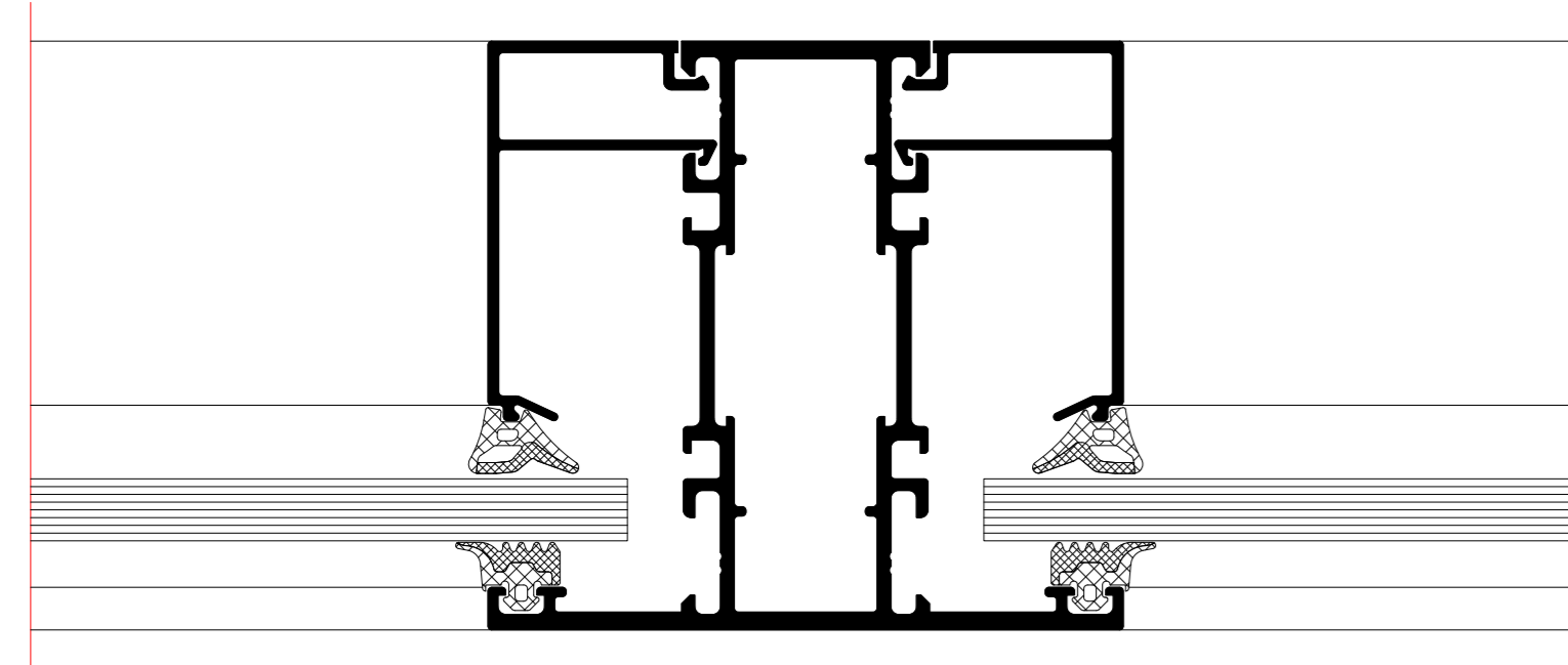
Riegel/Pfosten Riegel/Pfosten
