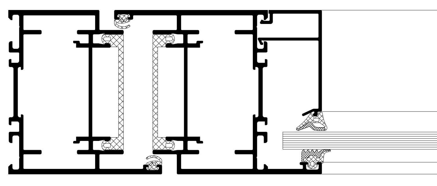
Flügelprofil Flügelprofil
